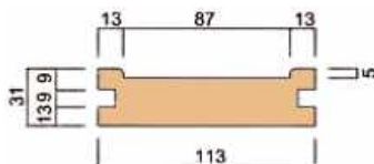
引違い縦枠
