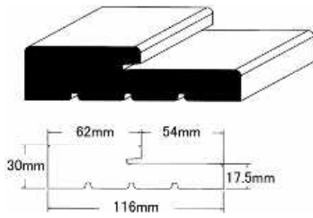
ドア枠
