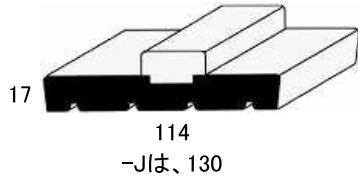
ドア枠
